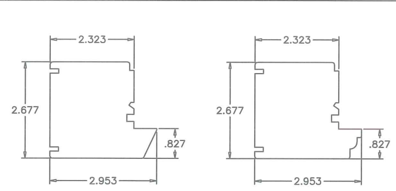
⑩ BOTTOM RAIL OPTIONAL
