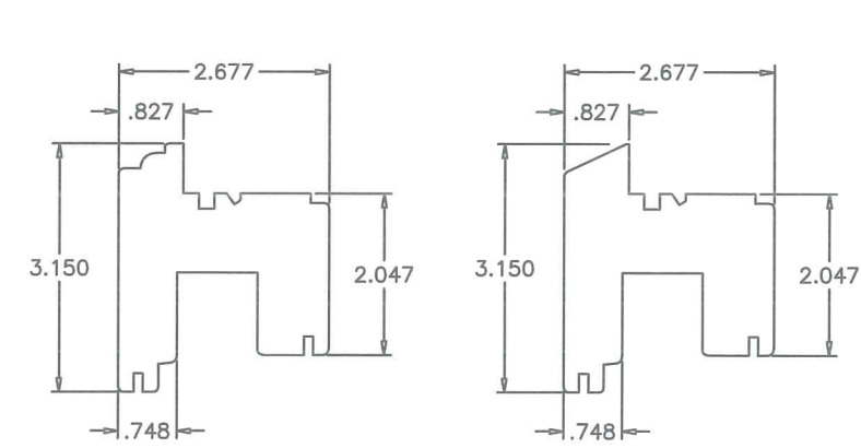
⑩ BOTTOM RAIL OPTIONAL
