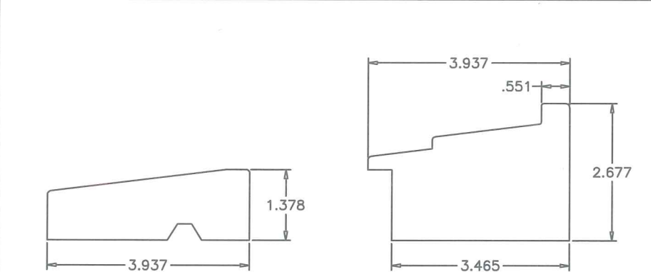
③ EXTERIOR FRAME JAMB ④ INTERIOR FRAME JAMB
